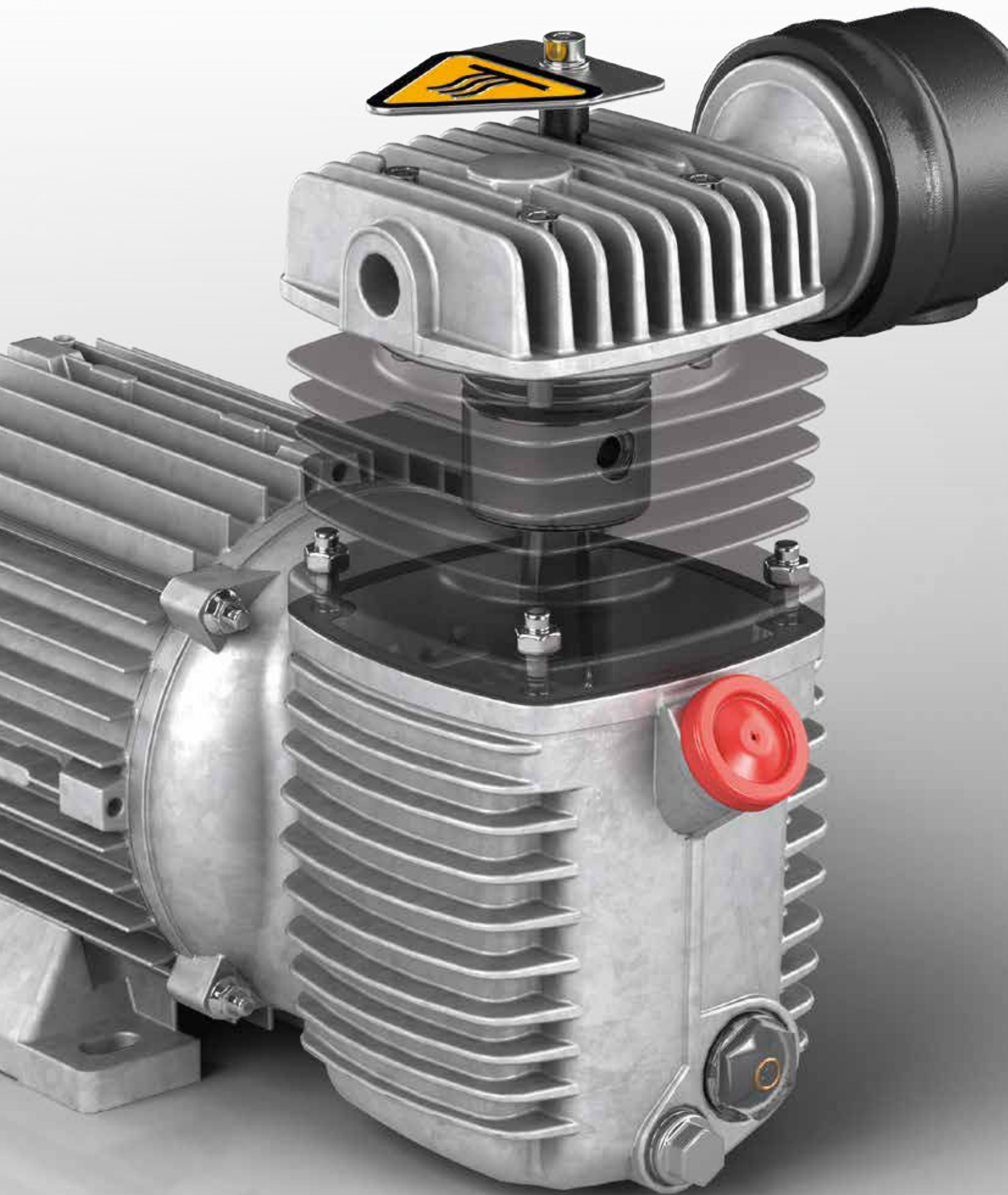
Рис.: Компрессорный блок CLASSIC
